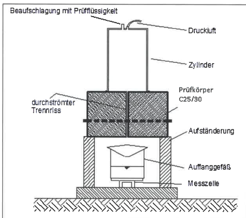
Abbildung 1: Schematischer Versuchsaufbau
